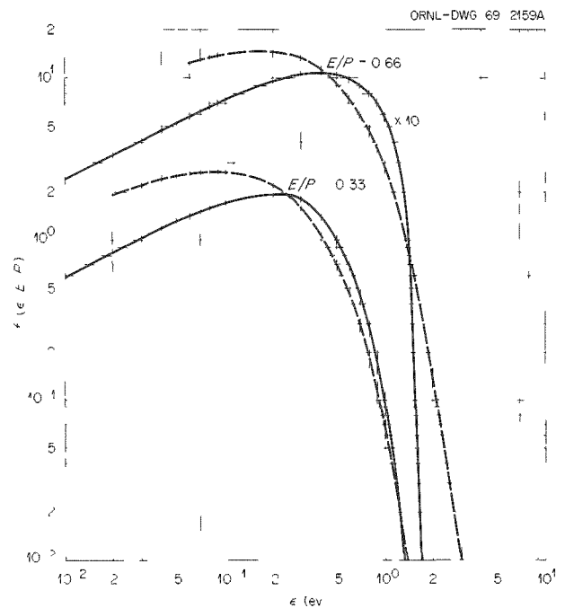
Fig. 16.4. Comparison of Distribution Functions in N_2 : Carleton and Megill 12 (---); Engelhardt et al 13 (—).
