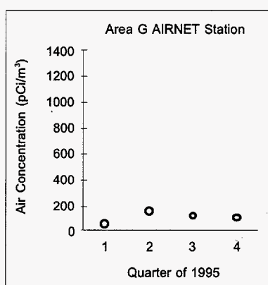
b. Plutonium-239
