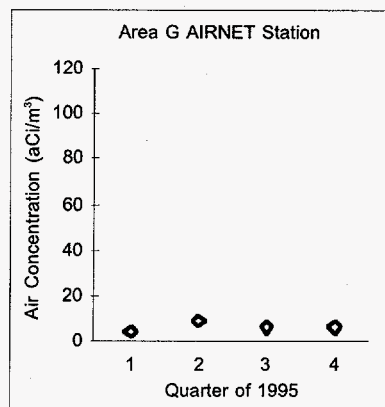
a. Plutonium-238
