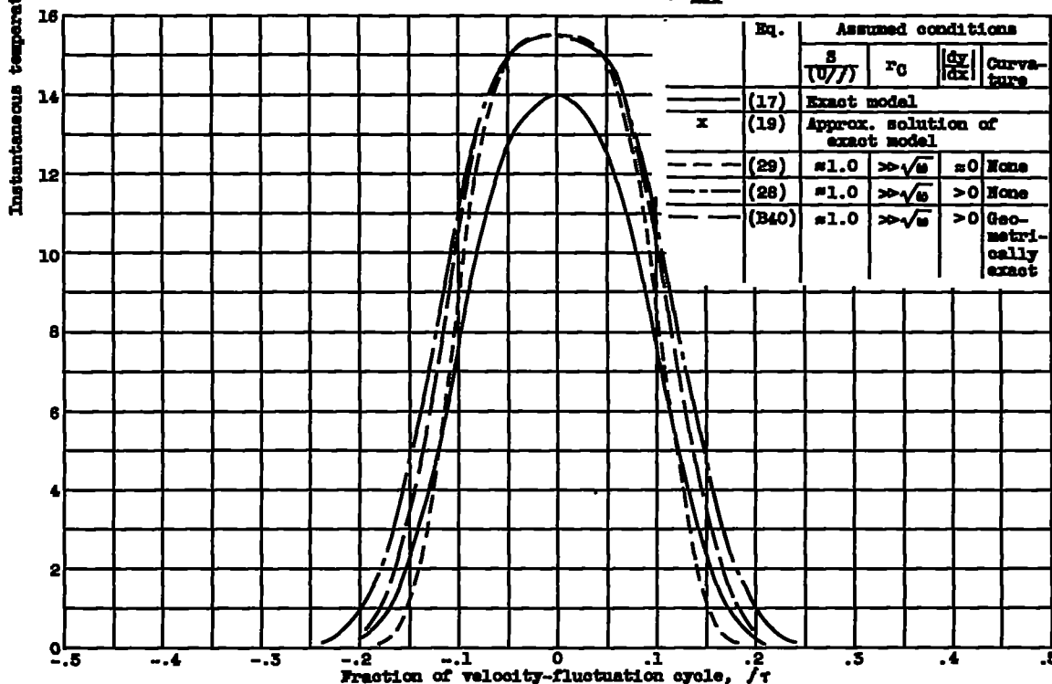
(d) Temperature-time variation at X/y_{max} = 1.0 .
