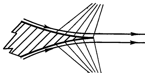
Inviscid S'(\alpha) = 0
