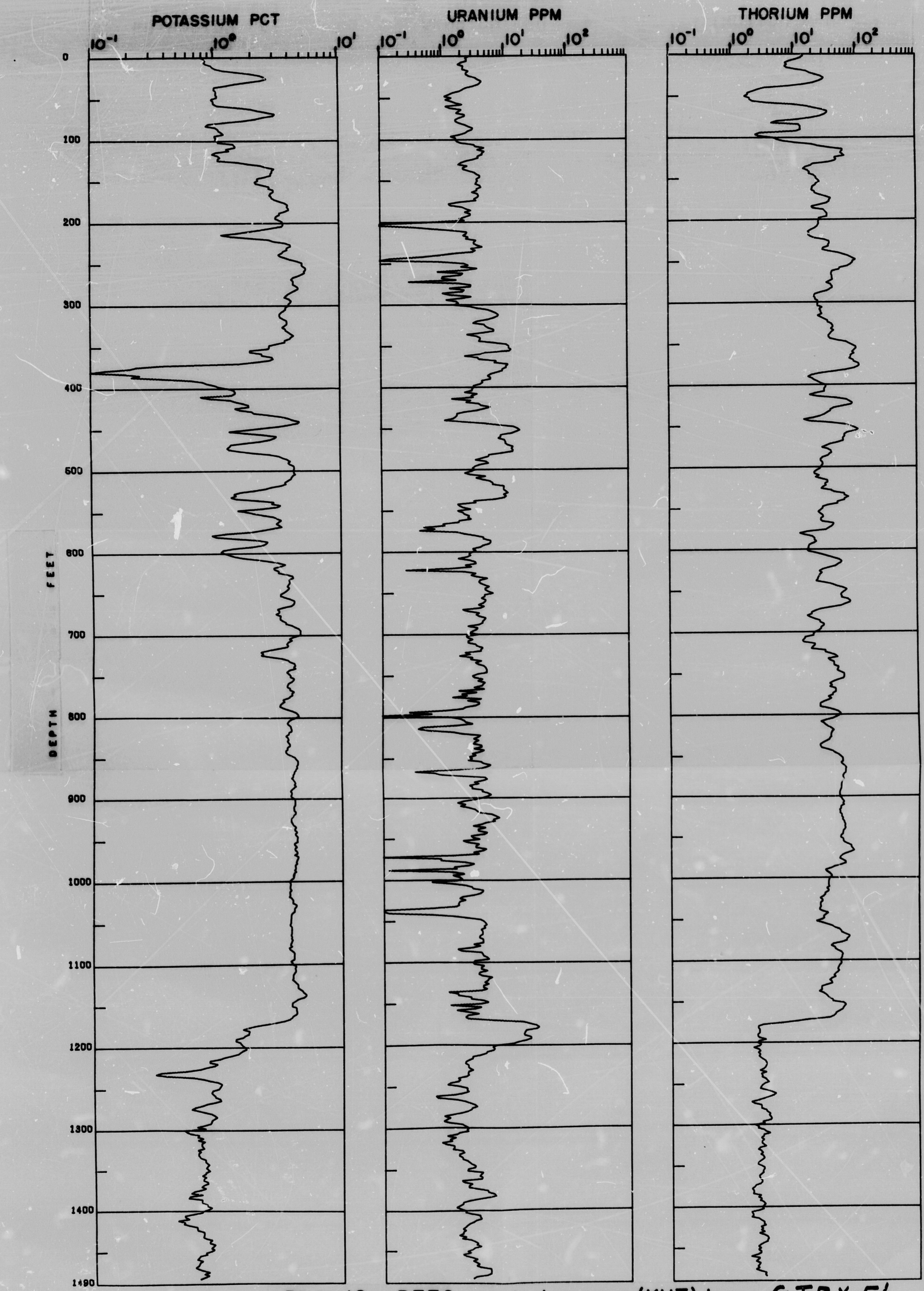
Plate 10. BFEC spectral gamma (KUT) log. GJBX-56
