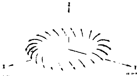
Fig. 3. Vorton.
