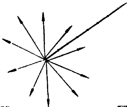
Fig. 1. Dirac monopole.
