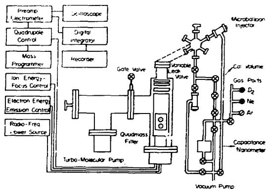
Fig. VII-9. Quadrupole mass spectrometer system.
