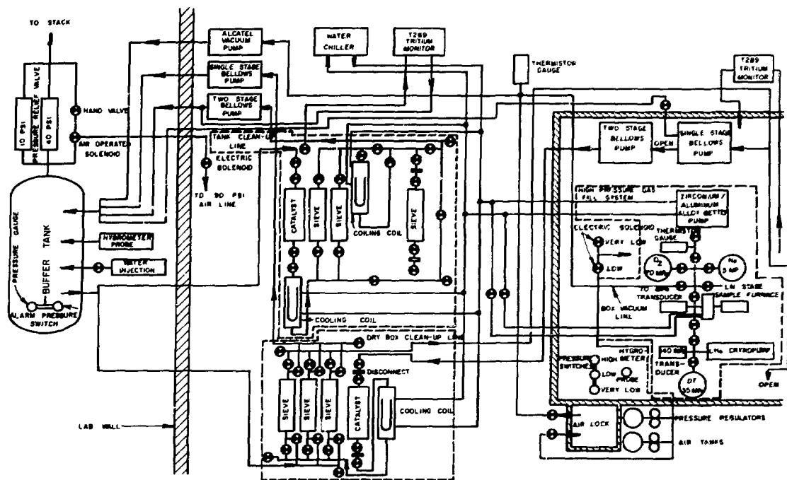
Fig. VII-7. Schematic of DT fill system.
