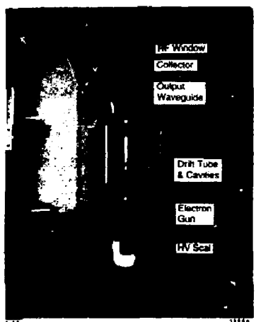
Fig. 1. The 67 MW production klystron.
