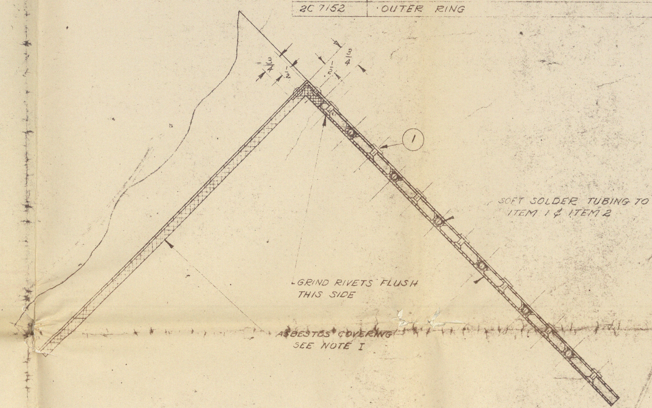
SECTION A-A
