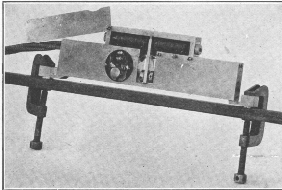
FIG. 50.— Electric telemeter
